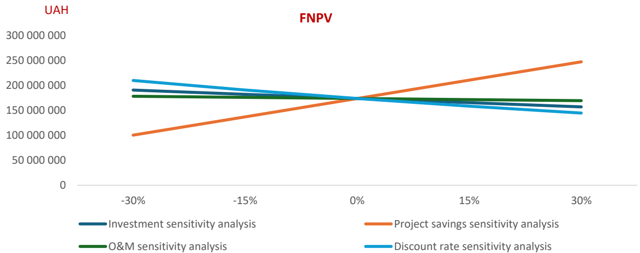
Рисунок2 . Профіль FNPV
